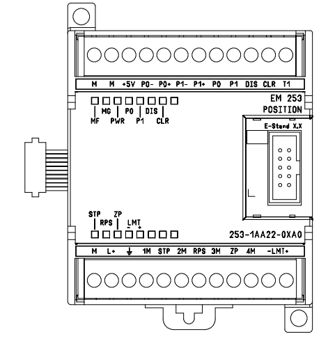
Bild 9-9 Positioniermodul EM 253
