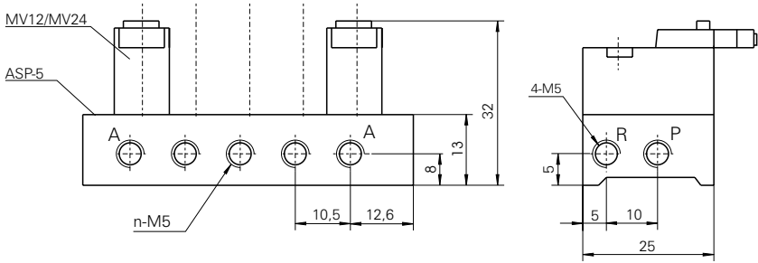
Mehrfachanschlussplatte (ASP-2...-10)
