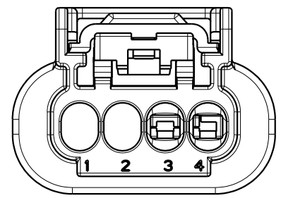
F150900 SCALE 2:1
