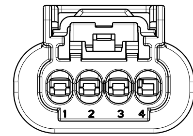
F250900 SCALE 2:1
