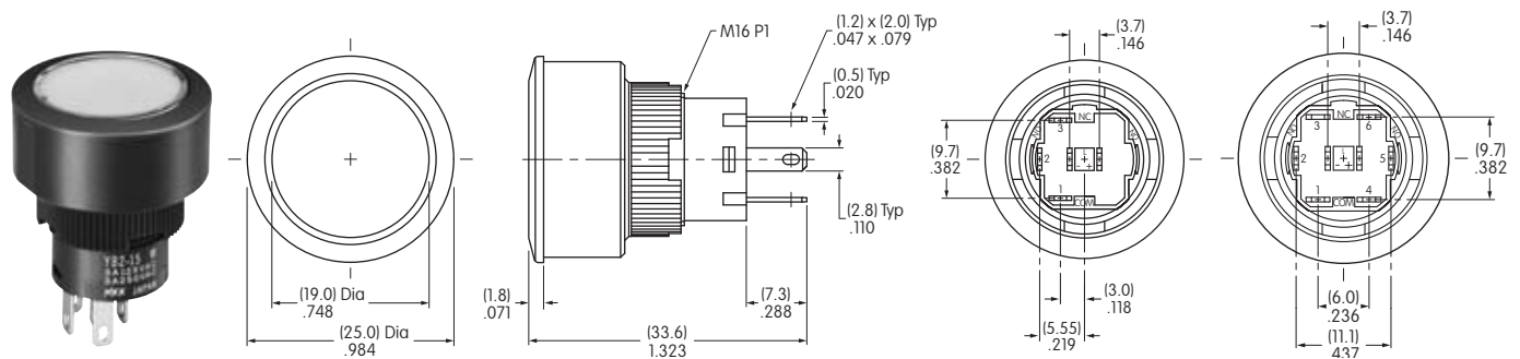
YB215CWCKW01-6B-JB
