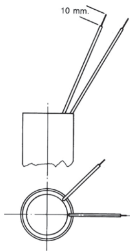
Fig. 6 Cavetti unipolari 0,5 mm 2 L = 150 mm
