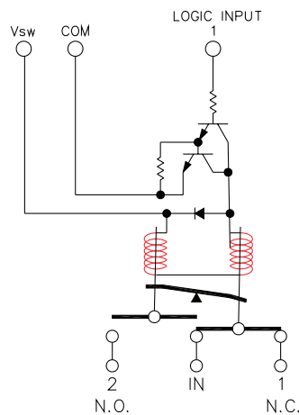
TTL
