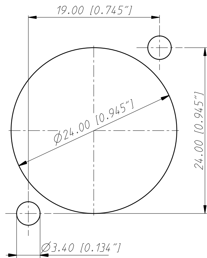
Print-Bohrplan (Bestückungsseite) PCB-Layout (component side)
