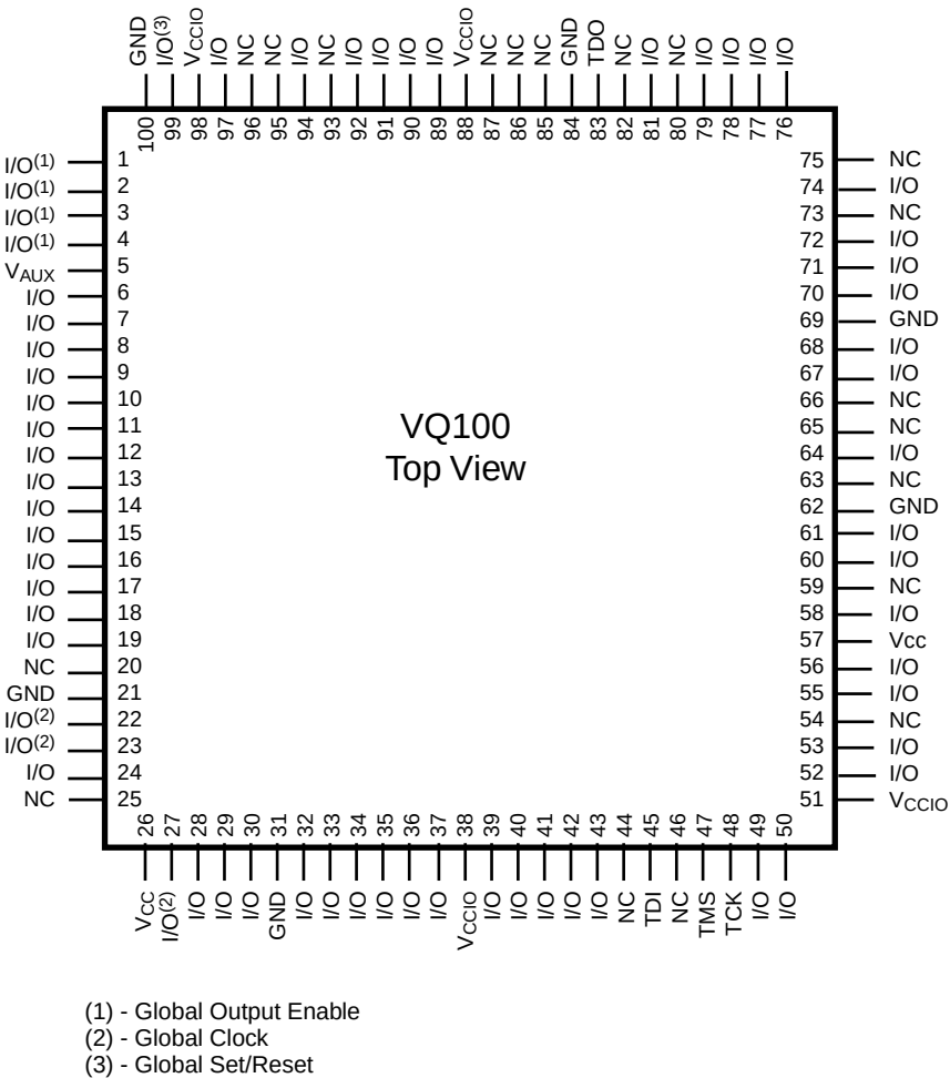
Figure 5: VQ100 Package
