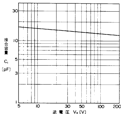
接合容量特性（代表特性） Junction Capacitance
