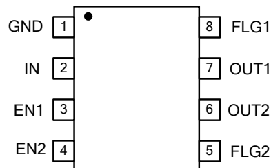
SO-8
