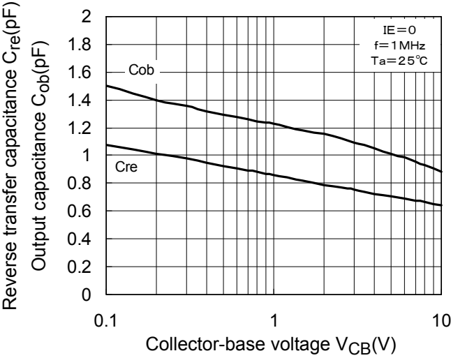
C_{re}, C_{ob}-V_{CB}
