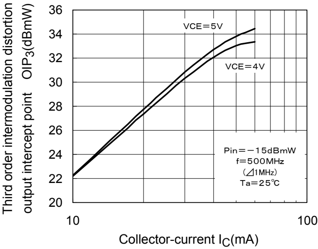
OIP_3-I_C
