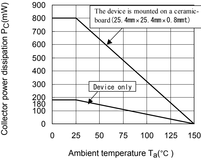
P_C-T_a
