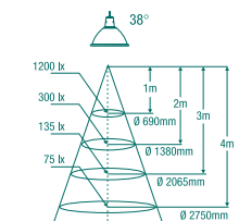
Dichroic 35W / 38°
