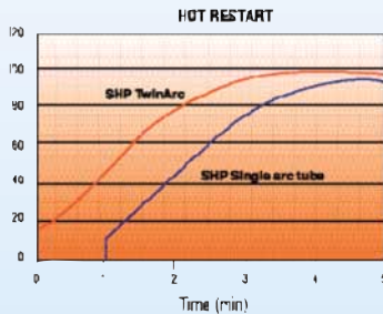
SHP-S TWINARC
