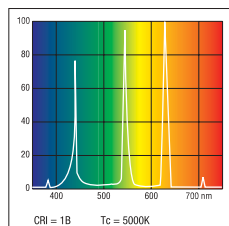
Daylightstar®
