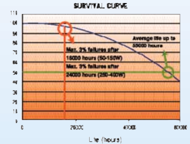
SHP-TS TWINARC
