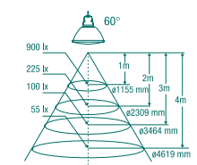
Coolfit 50W / 60°
