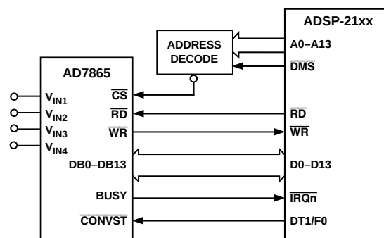
Figure 19. AD7865-ADSP-21xx Interface
