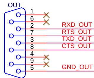
DB9_Male
