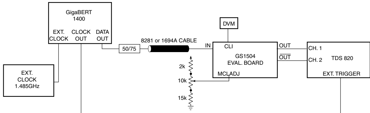
Fig. 1 Test Setup
