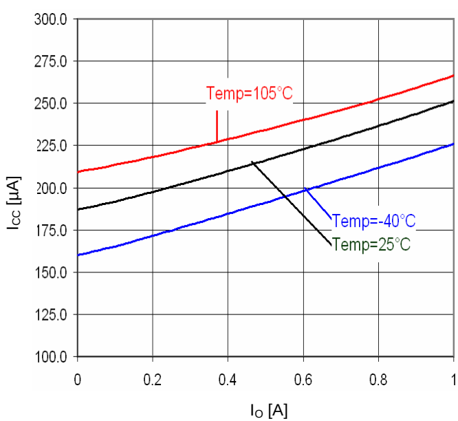
Fig.32 Io-Icc
