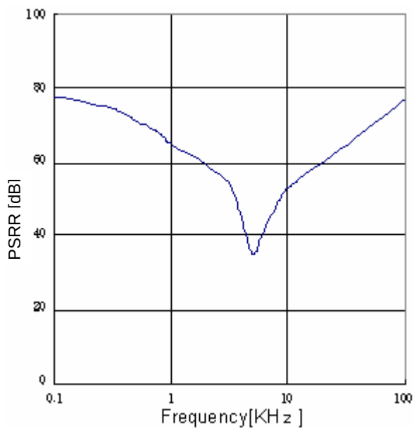
Fig.33 PSRR (Io=0mA)
