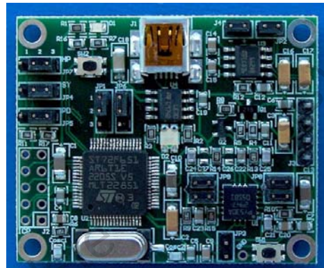
STEVAL-MKI037V1
