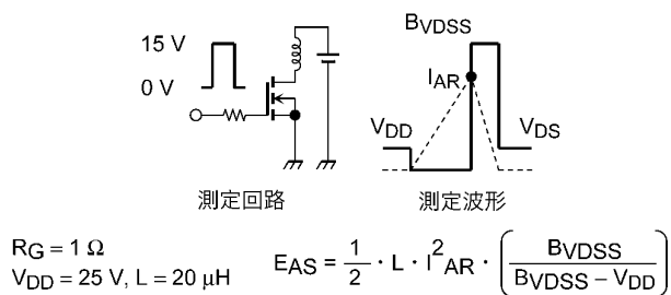
図 8.15 測定回路/測定波形
