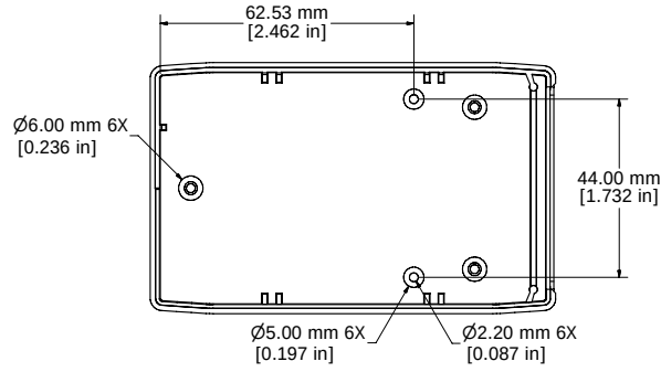
LID - INSIDE
