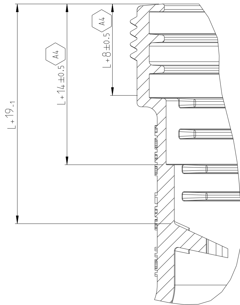
L+ = ADD LENGTH FOR CORRUGATED TUBE Zus. Länge des Wellrohrs
