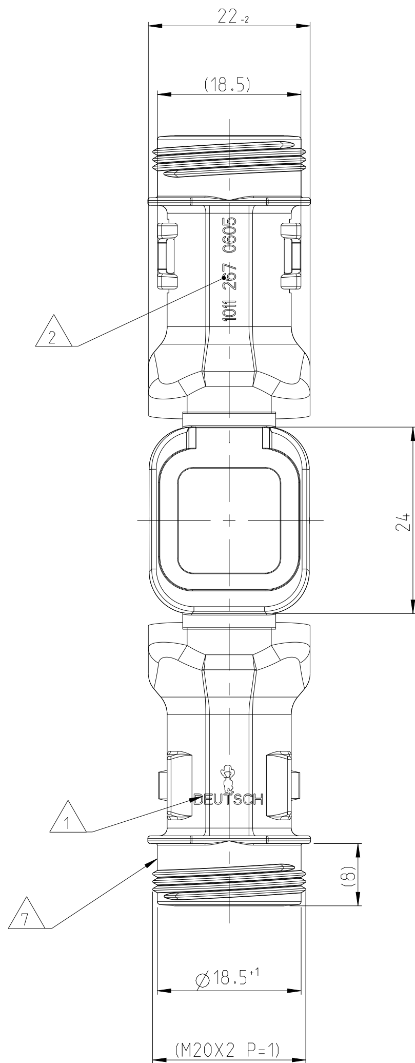
DELIVERY CONDITION AS SHOWN Lieferzustand wie gezeigt
