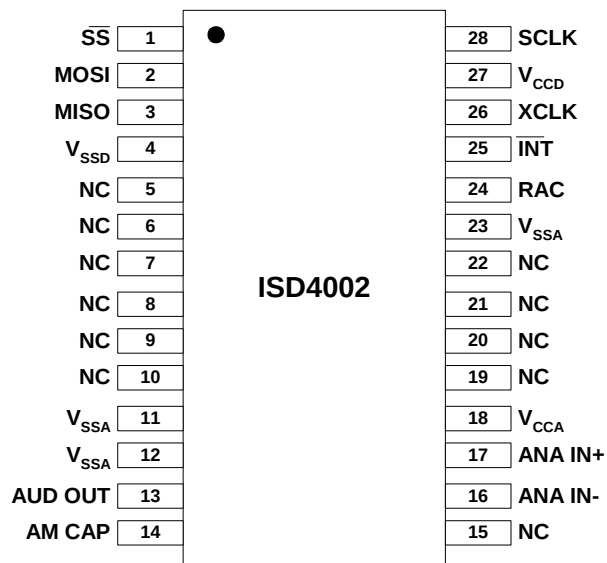
SOIC / PDIP
