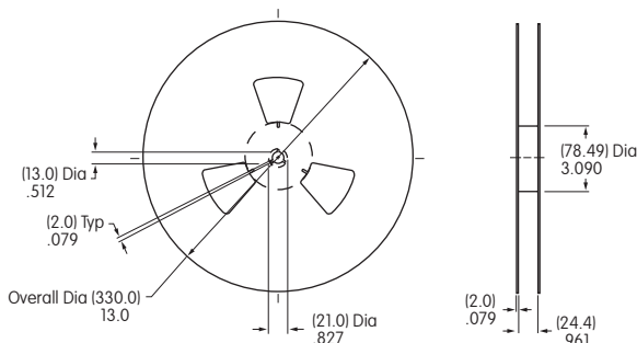
Reel Dimensions
