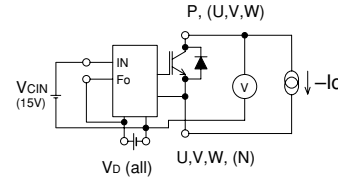
Fig. 2 V_{EC} Test
