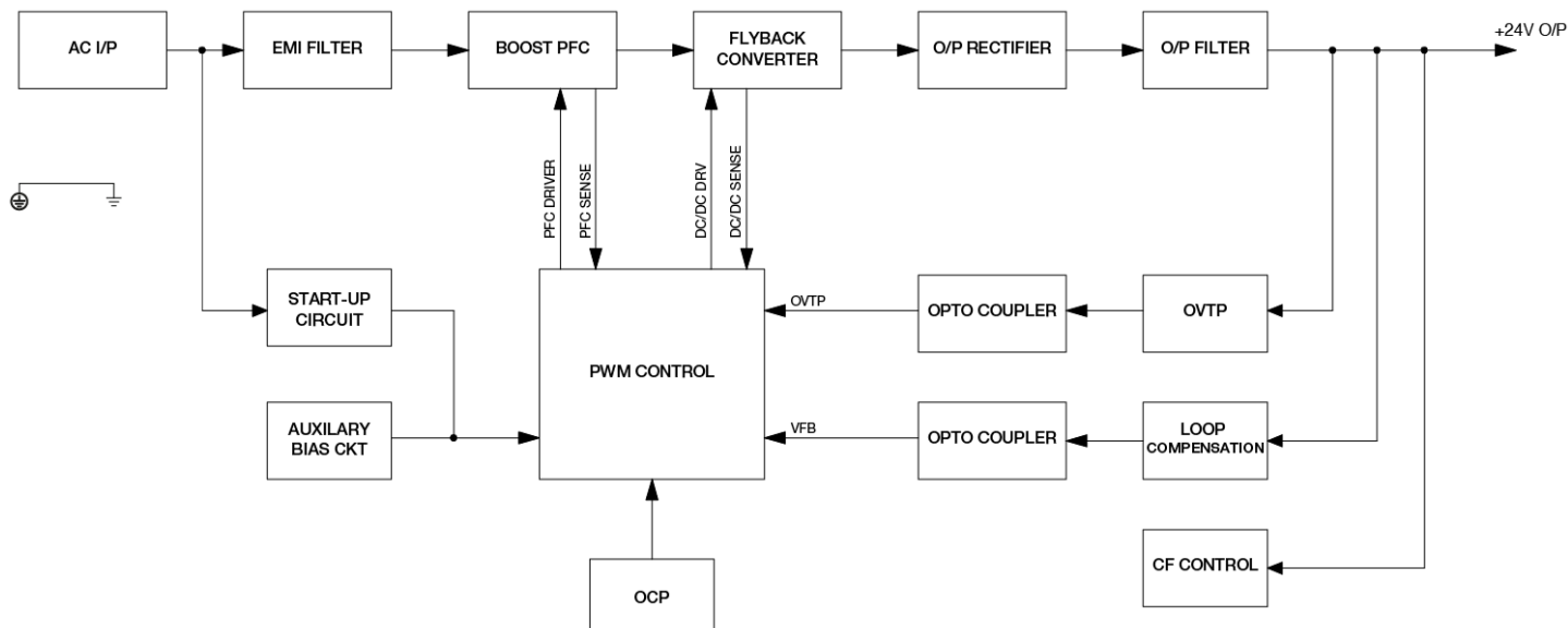
DRS-24V100W1□Z
