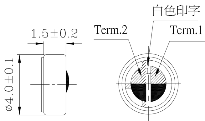
外觀尺寸圖
