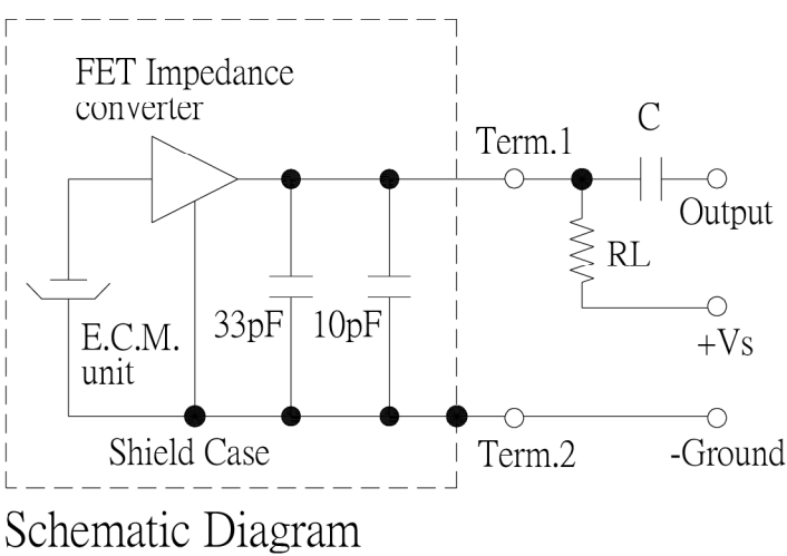
測量線路
