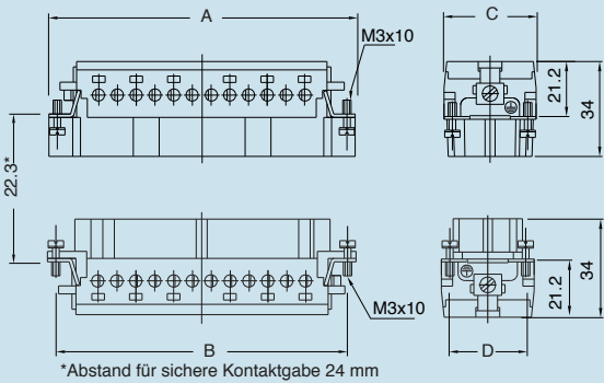
*Abstand für sichere Kontaktgabe 24 mm
