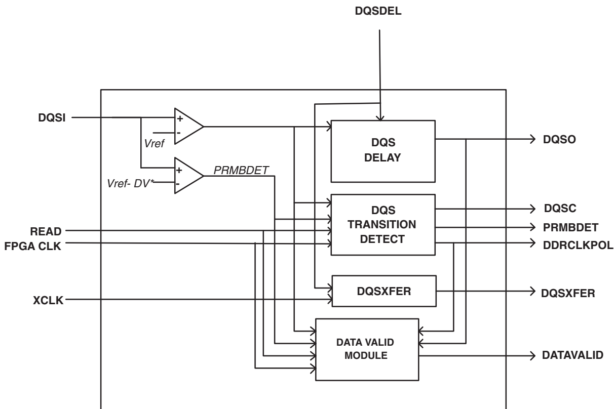
Figure 12-8. DQSBUFC Function
