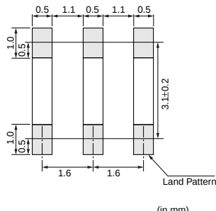
CSACV_X_Q
