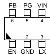
TSOT-23-6/SOT-23-6
