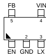
TSOT-23-5/SOT-23-5
