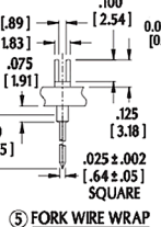
⑤ FORK WIRE WRAP
