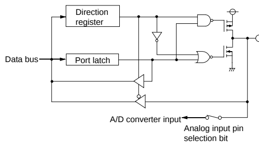
(13) Ports P20-P27
