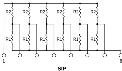
SIP
