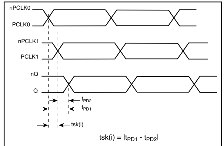
Input Skew
