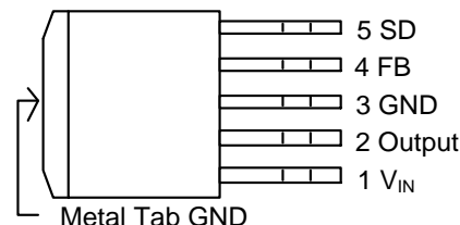
TO263-5
