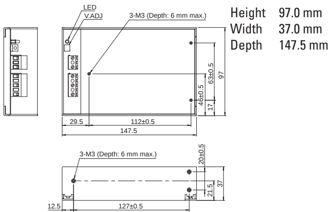
PS3L-D (50W)
