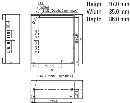
PS3L-A/B (10/15W)
