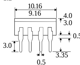
ISP845X ISP845
