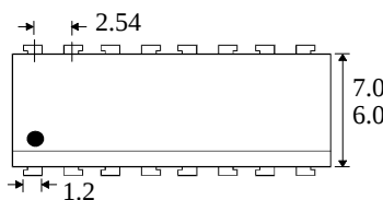
ISP845X ISP845
