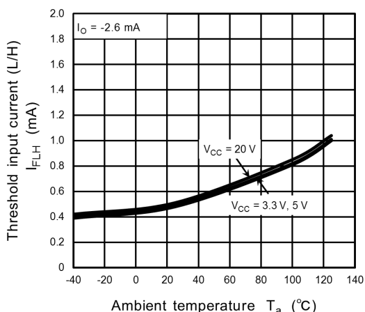
Fig. 12.2.11 I_{FLH} - T_a
