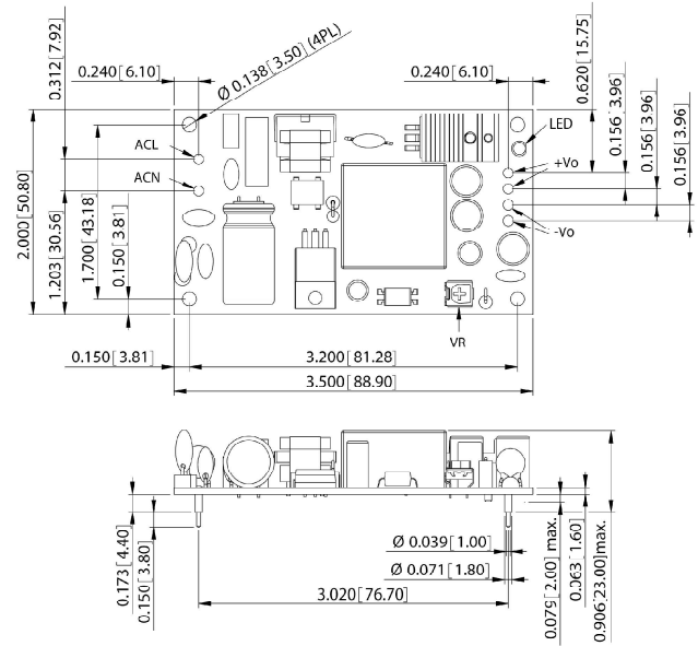
Outline Drawings (ZPSA20xx/P)
