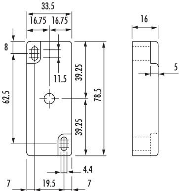
ACTUATOR S40
