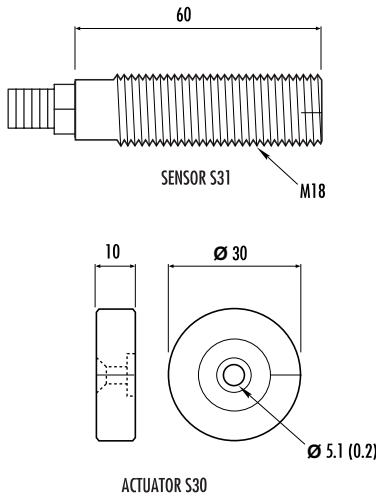
ACTUATOR S30
