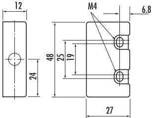
ACTUATOR - S10
