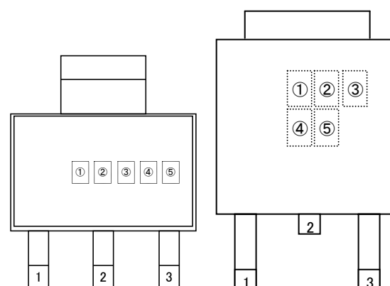
SOT-223
