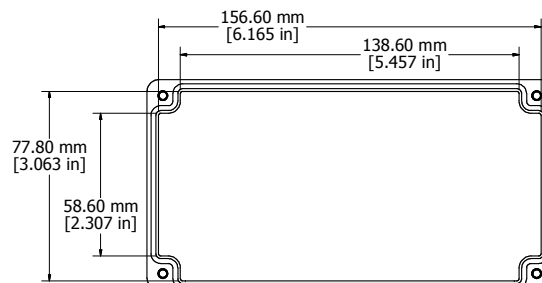
LID - INSIDE
