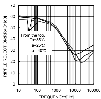
Fig.5 VO1 Ripple Rejection VO1 = 5V
