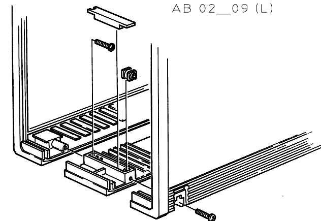
Montagezeichnung für AB 02_09 (L)
