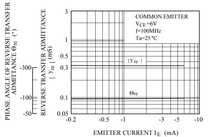
|y_{fe}|, \theta_{re} - I_E
