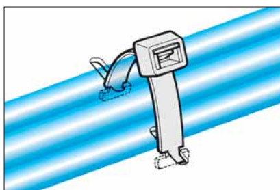
Het voetgedeelte van de CTF-serie is geschikt voor alle gangbare kabelgoten.
