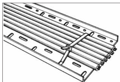
Fixeren van leidingen in een kabelgoot met de CTF-bundelband.
