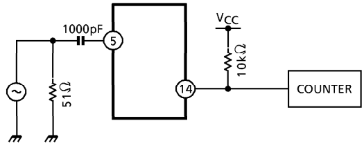
4. V_{TXIN} , V_{XIN}
