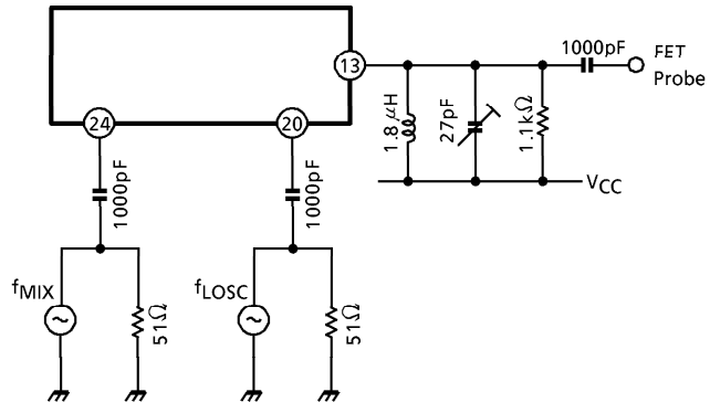
6. G_{VMIX}
