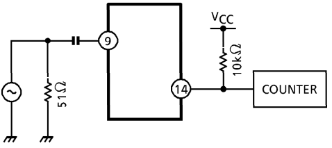
5. V_{XIN}
