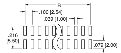
PH2-20-UA-SMT
