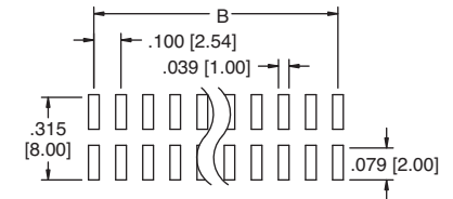
PH2-26-UA-SMT
