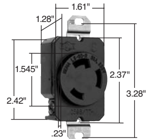
30A Receptacle
