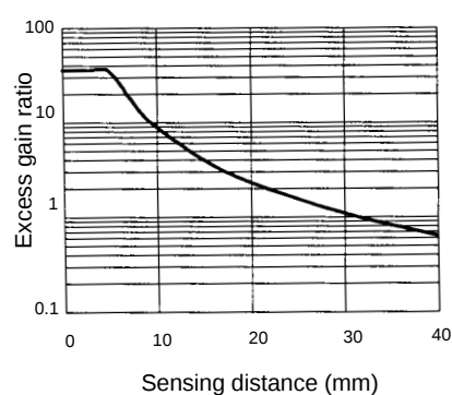
E32-D32 with E3JU-XR amplifier
