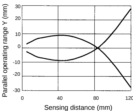
E32-DC200 with E3JU-XR amplifier
