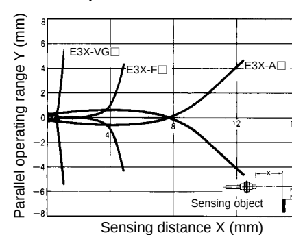
E32-D21 with E3X-A, E3X-F and E3X-VG amplifiers
