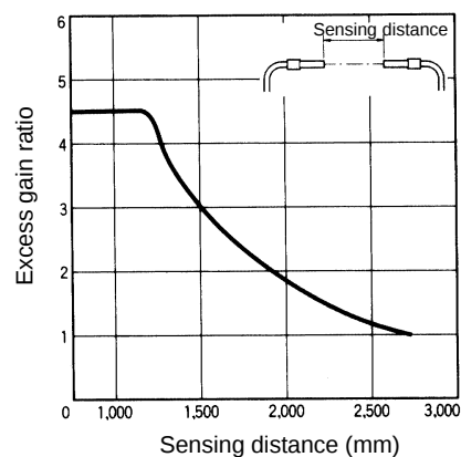
E32-T84S with E3X-NH amplifier
