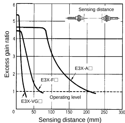
E32-T22L with E3X-A, E3X-F and E3X-VG amplifiers
