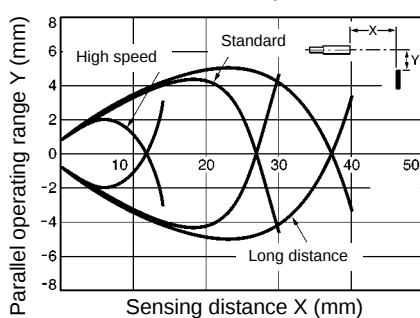
E32-DC200F with E3X-NH amplifier
