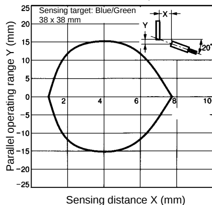
E32-D11L with E3X-A, E3X-F, and E3X-VG amplifiers
