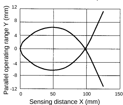
E32-UBDT1-3F with E3JU-X amplifier
