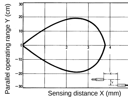
E32-T12F with E3X-NH amplifier
