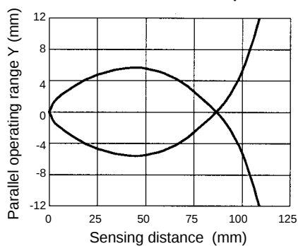
E32-UBDT1-6F with E3JU-X amplifier
