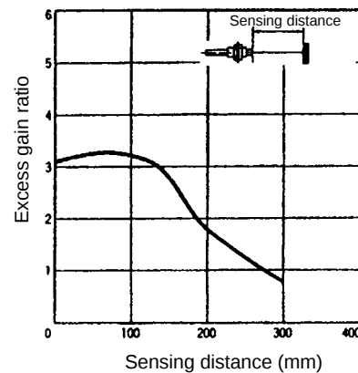
E32-DC200 with E3X-A11 amplifier
