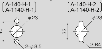
パネル穴明け寸法 Panel drilling dimensions
